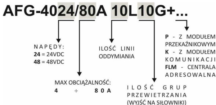
Rysunek 2. Oznaczenie typu, tabliczka znamionowa dla wersji AFG-4024, AFG-4048
