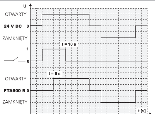
Schemat działania przekaźnika w FTA600 R
