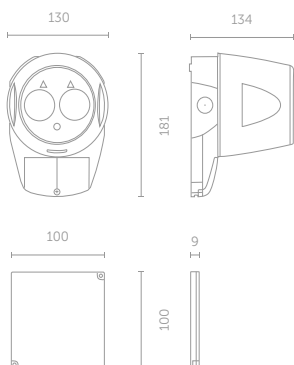
UCHWYT MONTAŻOWY OBUDOWY CZUJKI
