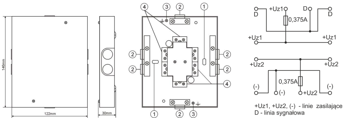
Rys.1. Widok puszek instalacyjnych i schemat połączeń.
