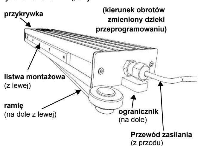
Rysunek 9: Siłownik „lewy”
