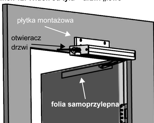
Rysunek 12: Widok od tyłu – drzwi „lewe”
