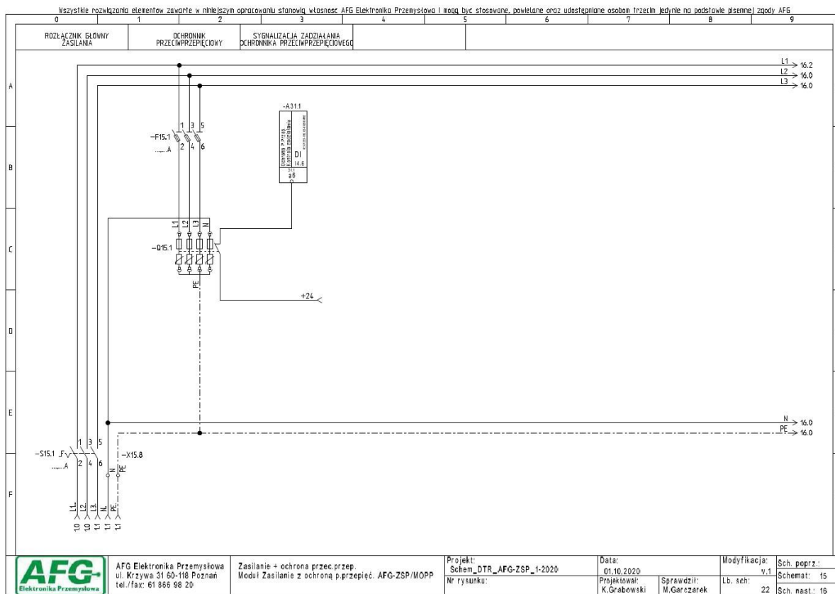
Rysunek 3.15. SCHEMAT MODUŁU ZABEZPIECZENIA PRZECIWPZEPĘCIOWEGO – AFG-ZSP/MOPP
