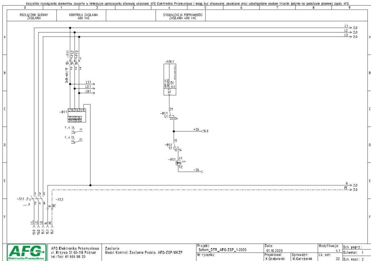
Rysunek 3.1. SCHEMAT MODUŁU KONTROLI i ZASILANIA – AFG-ZSP/MKZP
