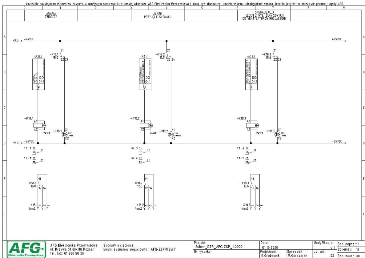
Rysunek 3.18. SCHEMAT MODUŁU SYGNAŁÓW WYJŚCIOWYCH – AFG-ZSP/MSWY
