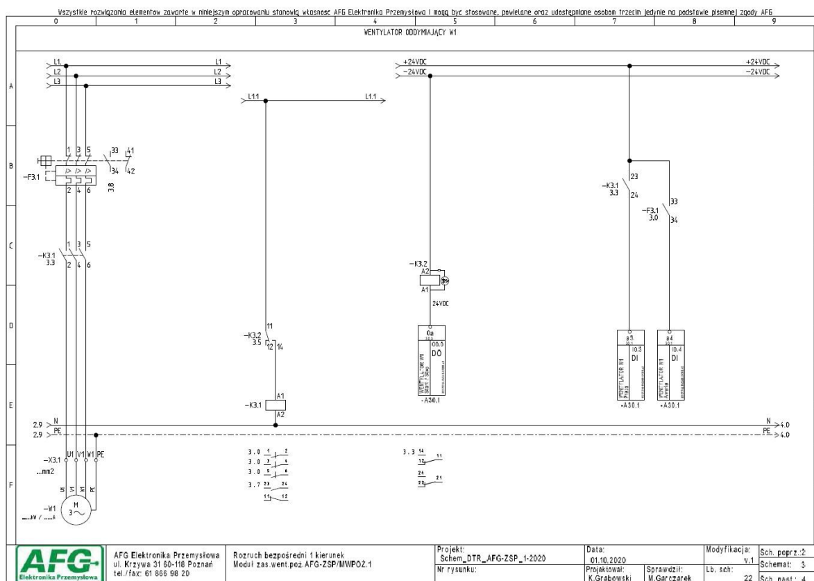
Rysunek 3.3. SCHEMAT MODUŁU ZASILANIA SILNIKA 3-FAZ JEDEN KIERUNKI - AFG-ZSP/MWPOŻ.1
