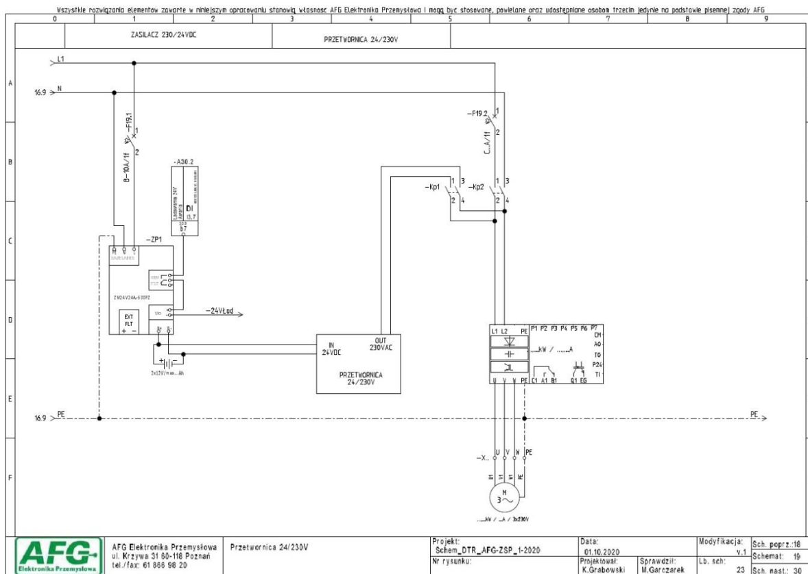
Rysunek 3.19. SCHEMAT MODUŁU PODTRZYMANIA 230V – AFG-ZSP/MP24-230
