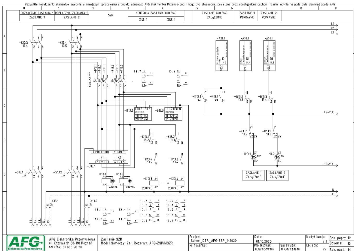
Rysunek 3.13. SCHEMAT MODUŁU SAMOCZYNNEGO ZAŁĄCZENIA REZERWY – AFG-ZSP/MSZR
