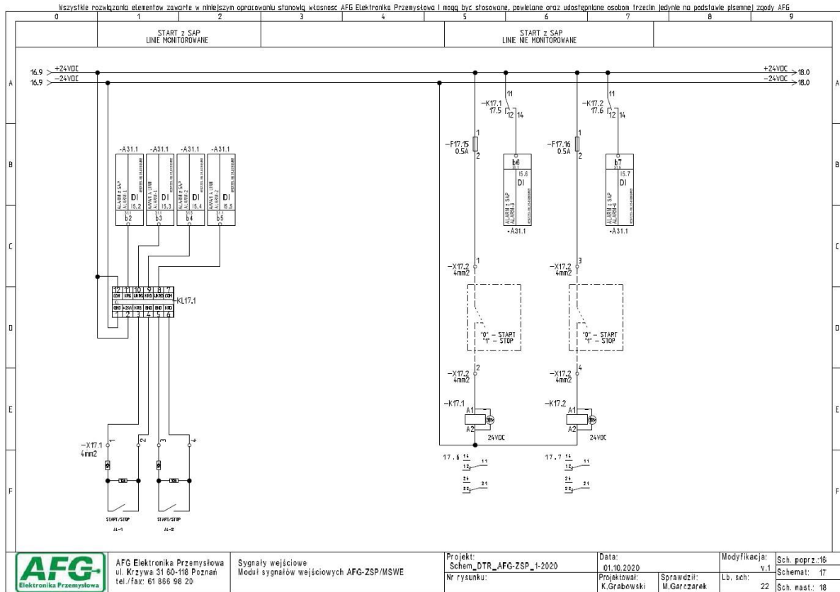
Rysunek 3.17. SCHEMAT MODUŁU SYGNAŁÓW WEJŚCIOWYCH – AFG-ZSP/MSWE
