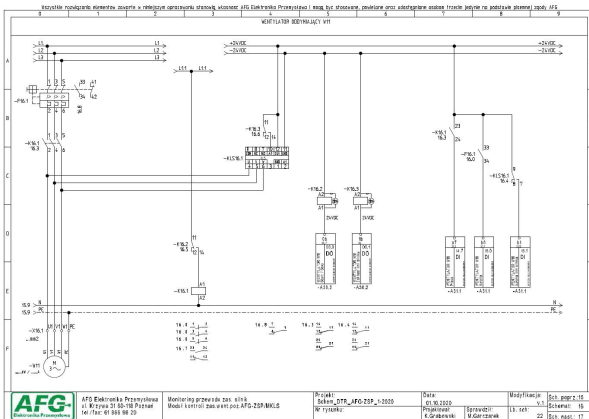
Rysunek 3.16. SCHEMAT MODUŁU KONTROLI CIĄGŁOŚCI LINII SILNIKA – AFG-ZSP/MKLS
