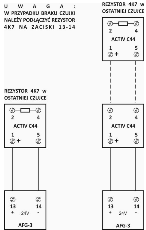
Rysunek 9. Podłączenie czujek typu Activ
