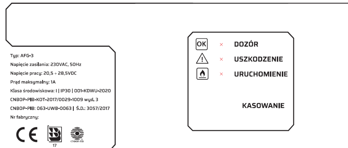
Rysunek 2. Panel sygnalizacyjno-kontrolny
