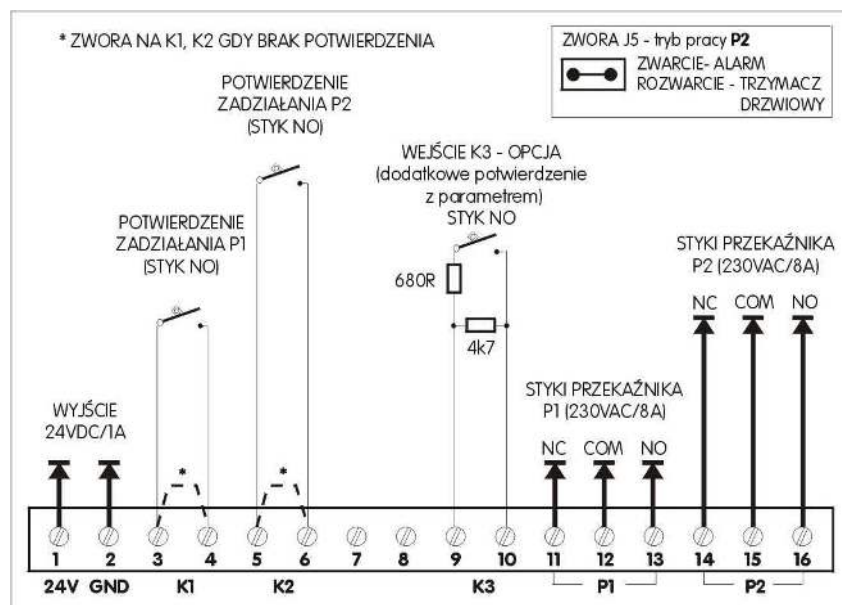
Rysunek 9. Schemat podłączenia modułu przekaźników pomocniczych AFG-2004P
