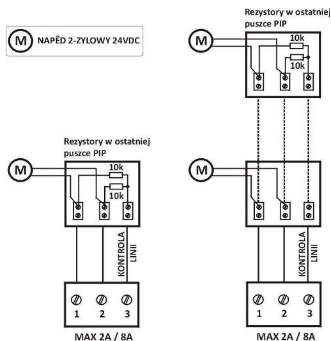
Rysunek 10. Wyście napędów: 2-żyłowe, kłapy i okna
