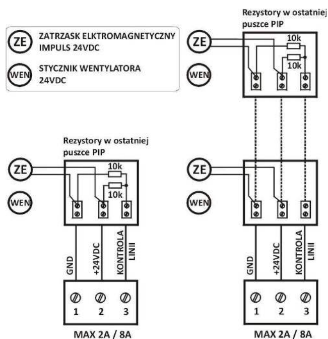
Rysunek 12. Wyście napędów: praca ZE lub WEN
