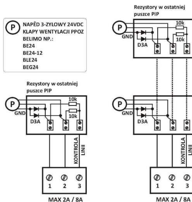
Rysunek 11. Wyście napędów: 3-żyłowe, kłap ppoz
